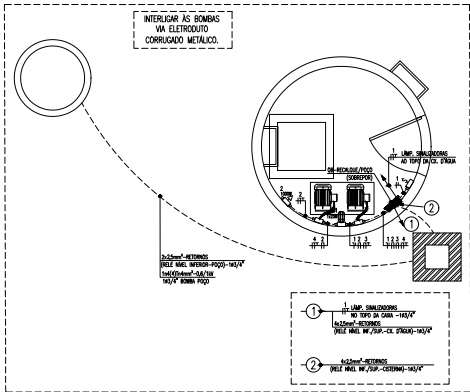
PLANTA BAIXA - CASTELO D'ÁGUA
